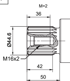
77 Estriado 21 Dentes
