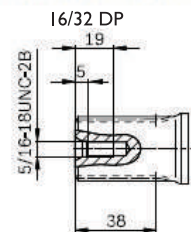
17 ESTRIADO 14 DENTES I2/24 DP
