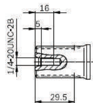
18 ESTRIADO 15 DENTES I6/32 DP
