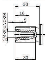
18X ESTRIADO 15 DENTES I6/32 DP
