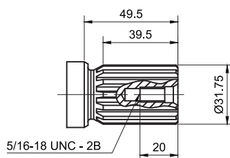
17X ESTRIADO 14 DENTES \varnothing 1\ 1/4"
