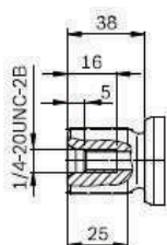
18X ESTRIADO 15 DENTES I6/32 DP
