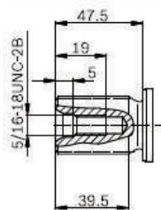
17X EIXO ESTRIADO 14 DENTES 12/24 DP
