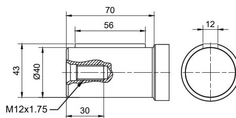
41 Cilindro Chavetado ø40mm
