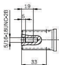
17 ESTRIADO 14 DENTES 12/24 DP
