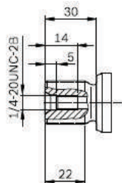
09X ESTRIADO 11 DENTES I6/32 DP
