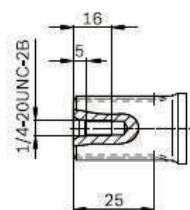
13 ESTRIADO 13 DENTES I6/32 DP
