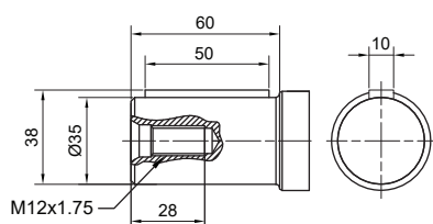
40 Cilindro Chavetado ø35mm
