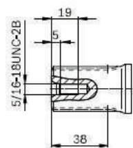
17 EIXO ESTRIADO 14 DENTES 12/24 DP
