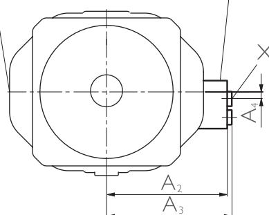
Montagem da válvula de pilotagem para sentido de rotação à esquerda
