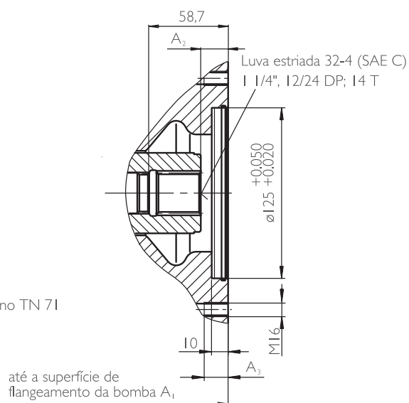
Corte A - B
