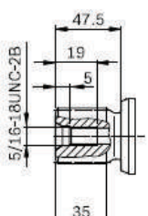
17X ESTRIADO 14 DENTES 12/24 DP
