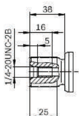
18X EIXO ESTRIADO 15 DENTES 16/32 DP
